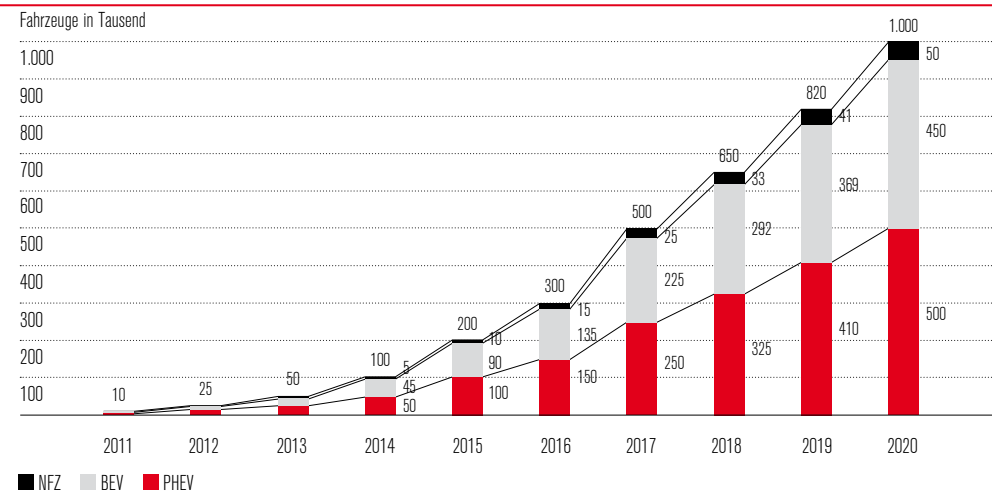
Abbildung 10: Abgestimmte Markthochlaufkurve
